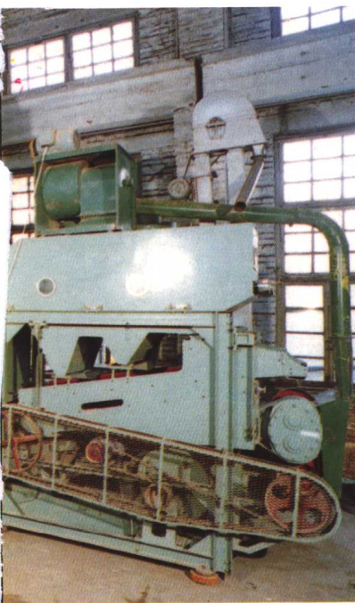
▲ 机械制造厂精米 联合加工设备
