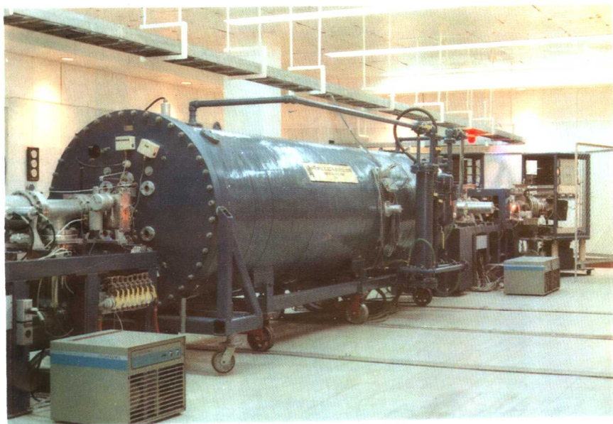
复旦大学 2 \times 3\text{MV} 串列加速器外貌 (见正文第四章)
