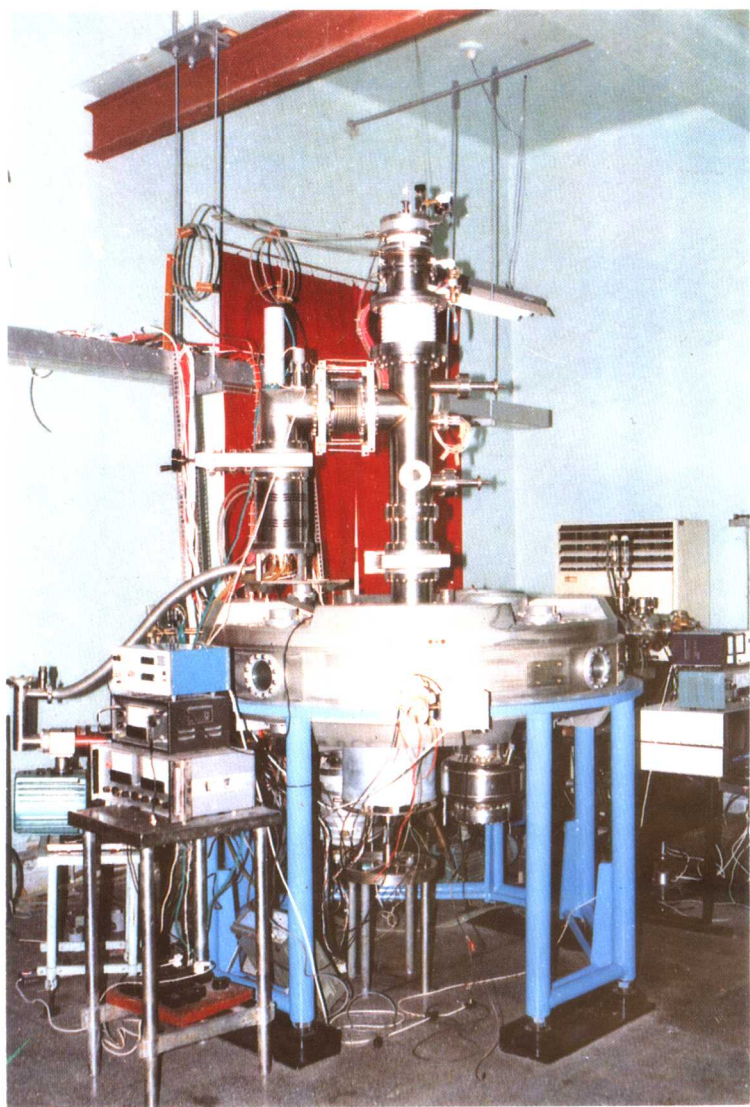
小型回旋加速器质谱计的外型照片（见正文第六章）
