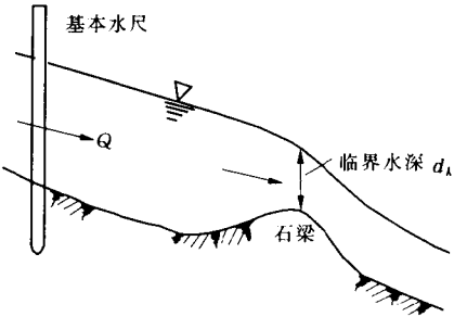
图 1-1 低水石梁控制示意
