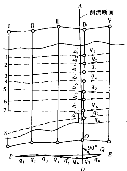
图 1-3 水流平面
