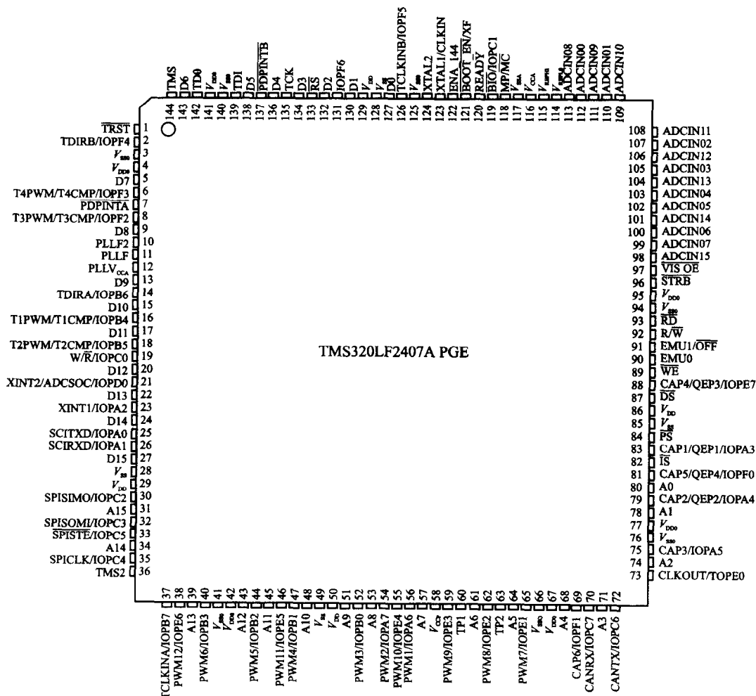
图 1-1 TMS320LF2407A 封装
