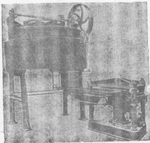
第六圖 英美式油粕蒸熱器與油餅型製機 (左蒸熱器，右型製機)
