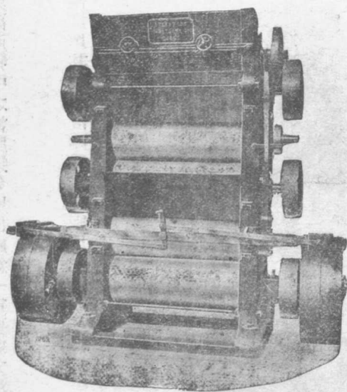
第一圖 英美式種子碾碎機
