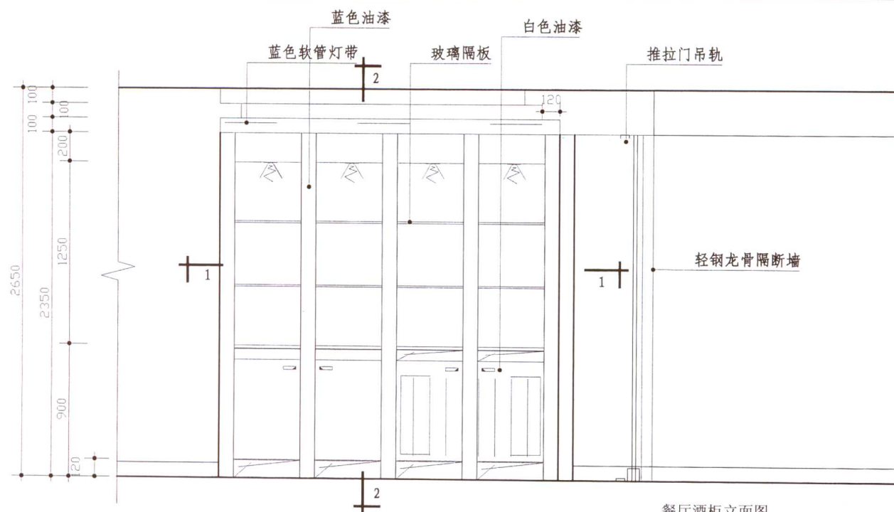
餐厅酒柜立面图
