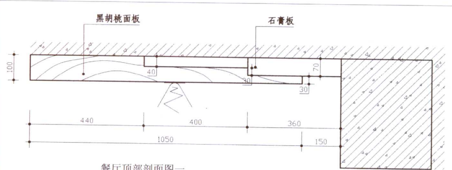
餐厅顶部剖面图一
