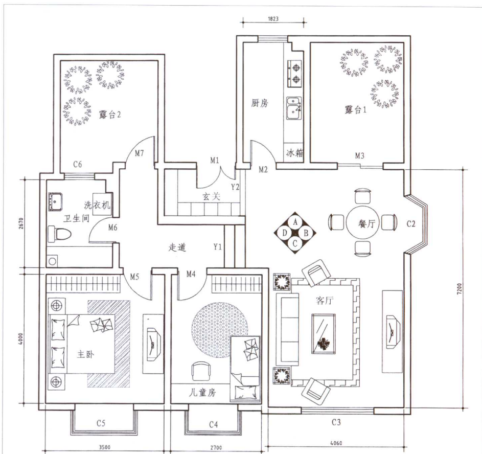
平面图
