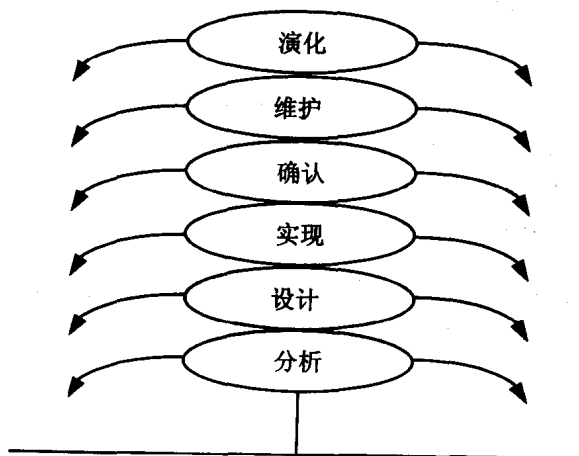
图 1.4 喷泉模型
