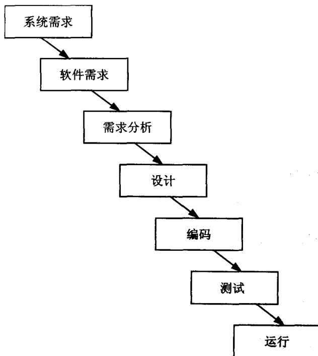
图 1.3 瀑布模型
