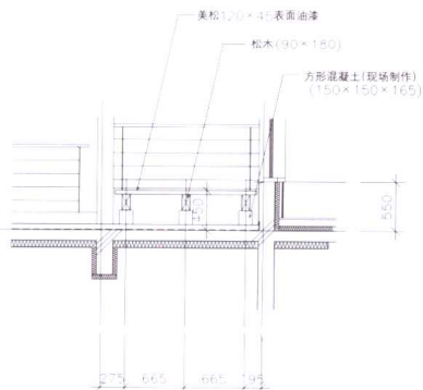
B断面详图(露台)
