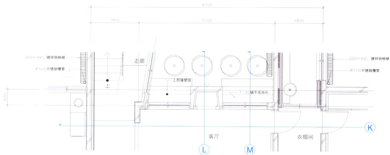
一层客厅平面详图(竹林庭院)
