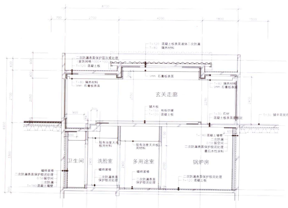
玄关、走廊剖面详图-I部分
