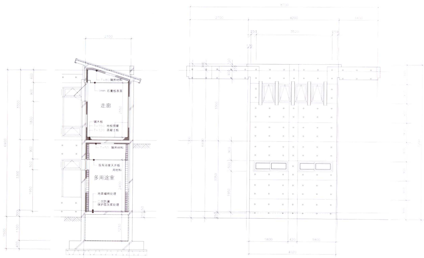
玄关、走廊剖面详图-J部分
