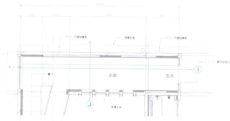
玄关平面详图
