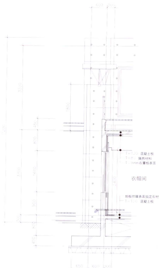
外壁剖面详图 - D部分
