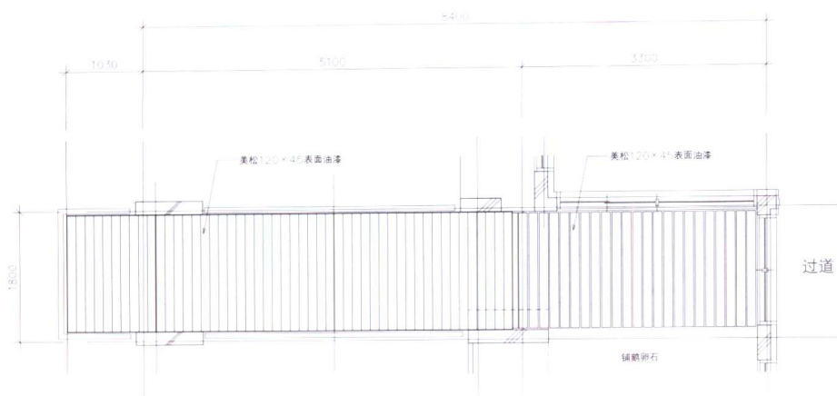
露台平面图(桥的部分)
