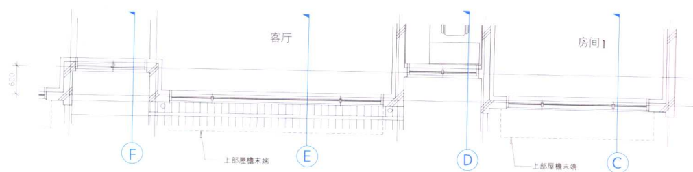
一层客厅平面详图(客厅天棚、阳台部分)
