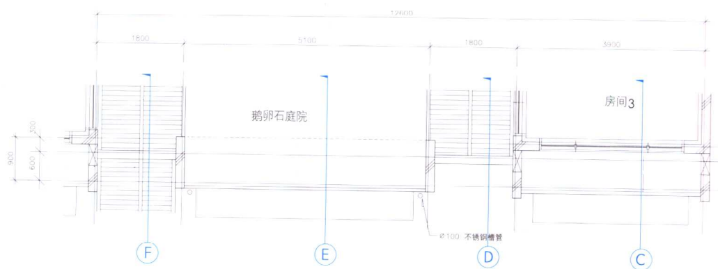
二层阳台平面详图
