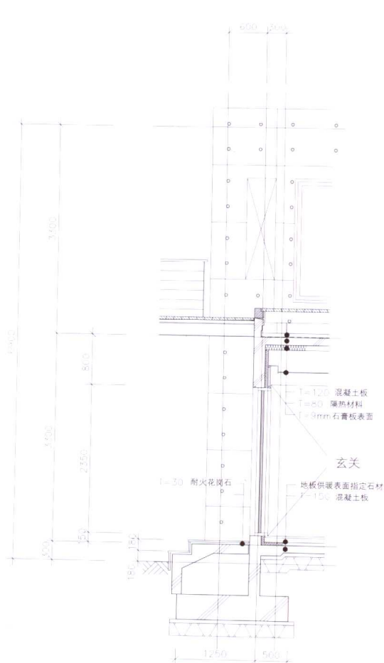
玄关外壁剖面详图(一楼客厅玄关部分) - F部分
