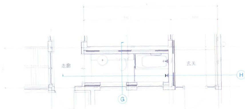
二层卫生间平面详图
