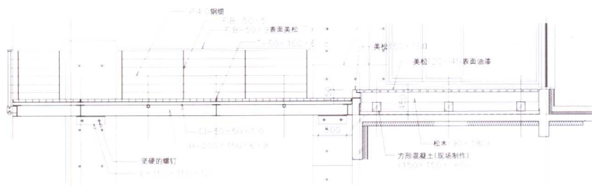
露台构造剖面图(桥的部分)
