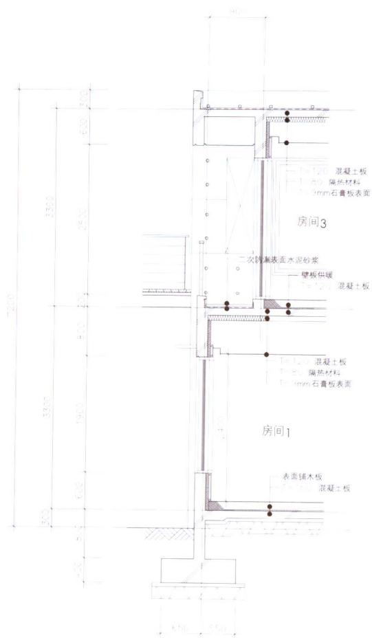
房间1外壁剖面详图(玻璃天棚部分) - C部分
