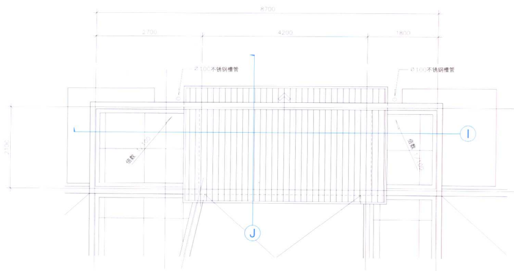
玄关屋顶层平面详图
