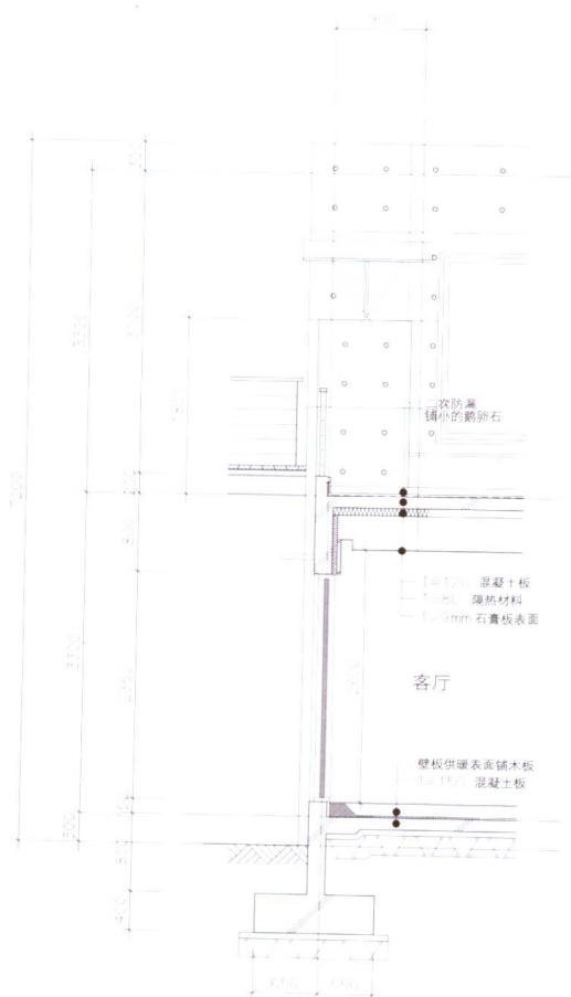
客厅外壁剖面详图 - E部分
