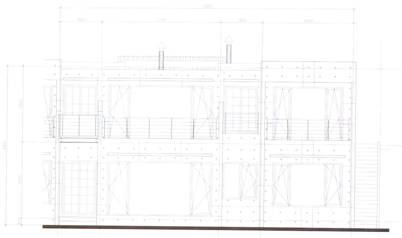
正面详图
