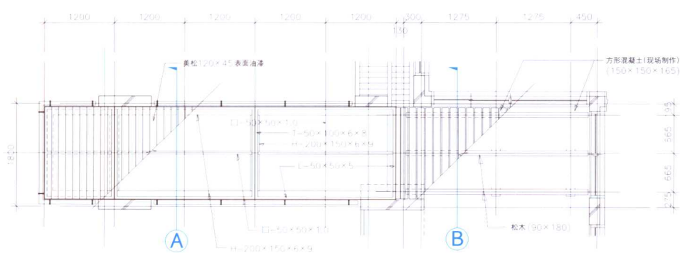
露台构造平面图(桥+露台)
