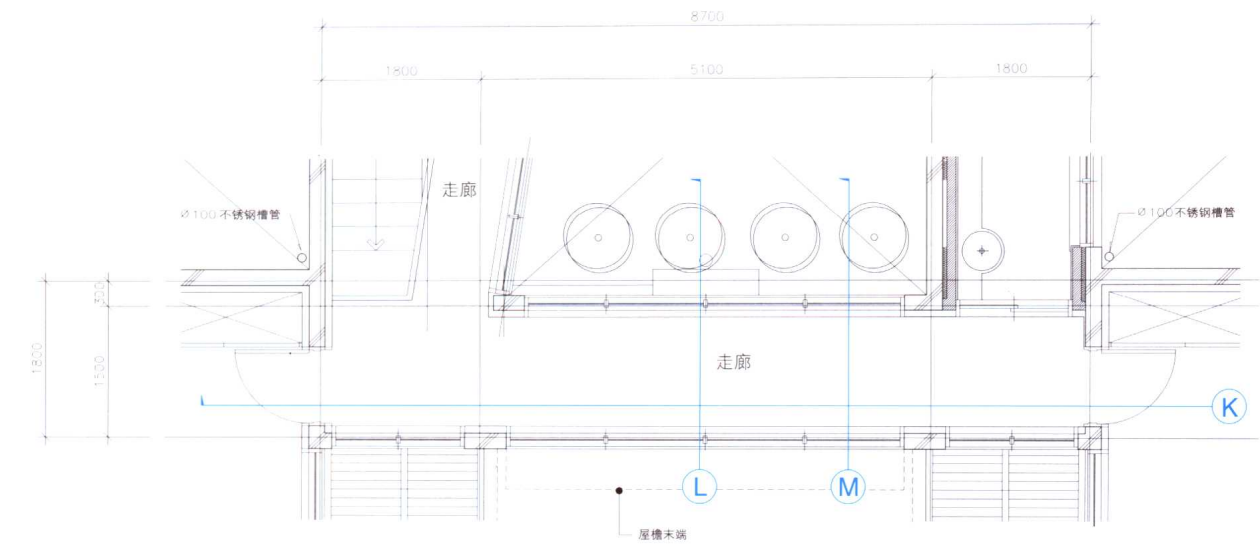
二层走廊平面详图
