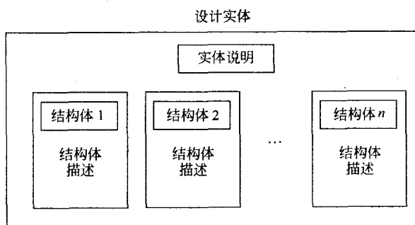
图 2.2 VHDL 程序的基本组成
