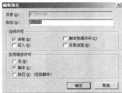
图8 【编辑别名】对话框
