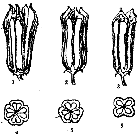
图6 蒴果类型
