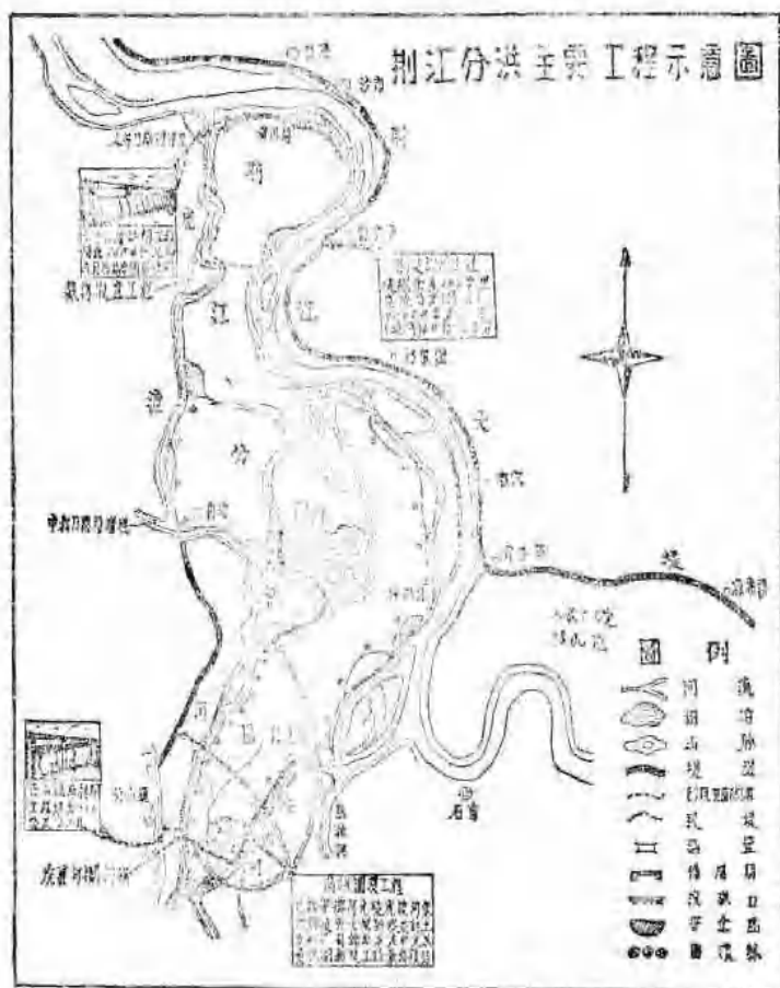
荆江分洪主要工程示意圖
