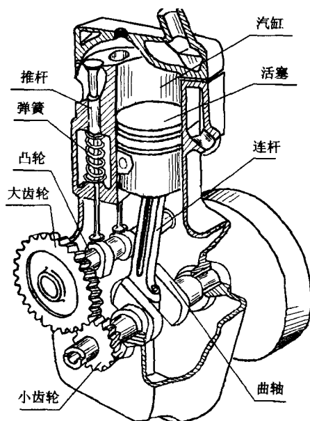
图1-1 内燃机
