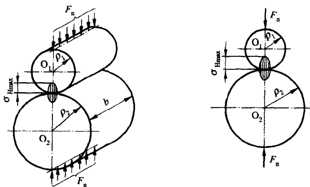
图 1-3 两个圆柱体的接触应力
