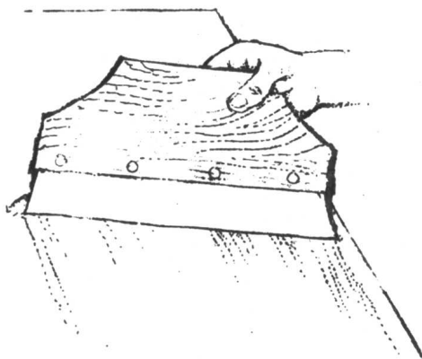
图 1-11 刮胶示意图
