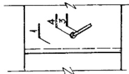
双扇门配电箱把手连门门正面剖面图 1:10
