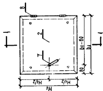
单扇门正面图
