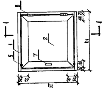
单扇门正面图
