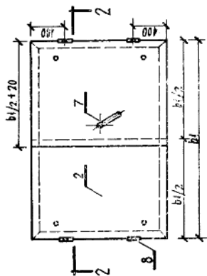
双扇门正面图
