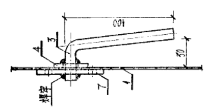
把手在箱门上的安装 1:2
