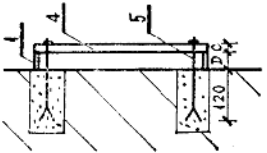
1-1剖面图
