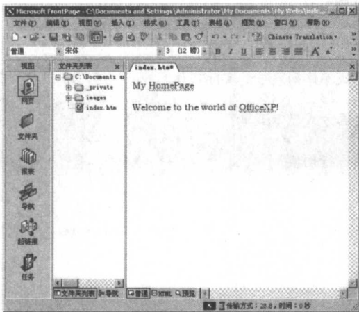
图 2.1 网页项目
