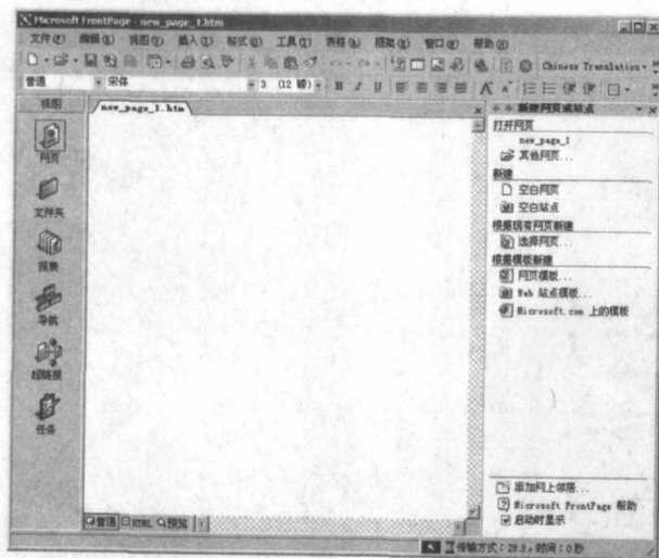
图 1.1 FrontPage 界面
