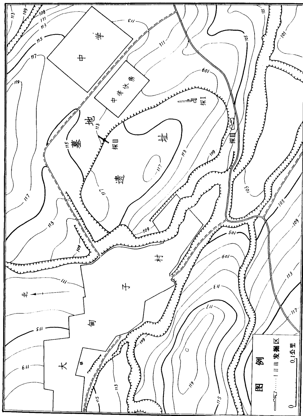
图二 大甸子遗址、墓地地形图
