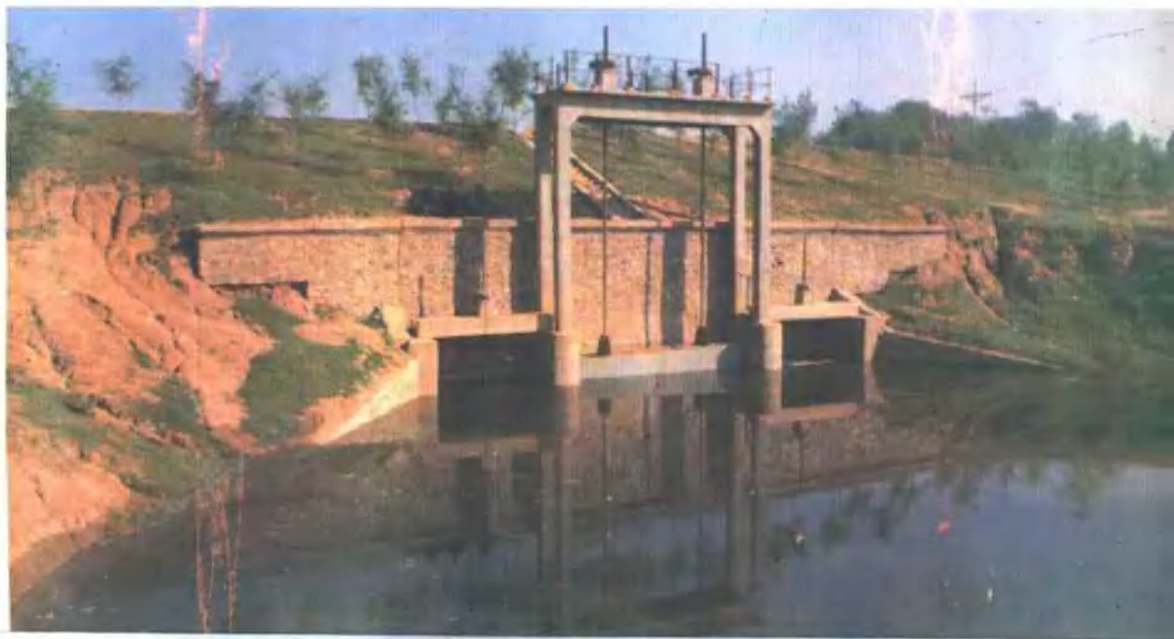
▼ 漳河左堤岸上防洪闸
