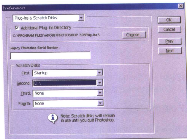
图1-5 设置临时盘
