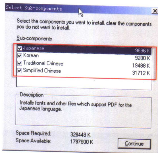
图 1-3 Sub-components 菜单
