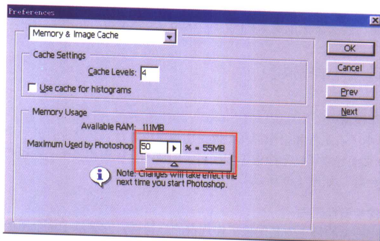
图 1-4 分配内存
