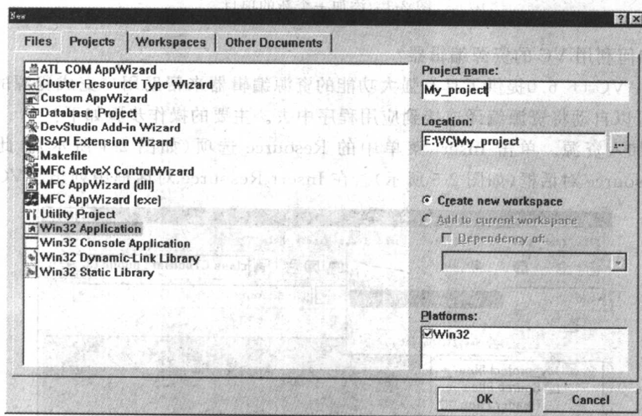
图 2-2 Project 选项卡
