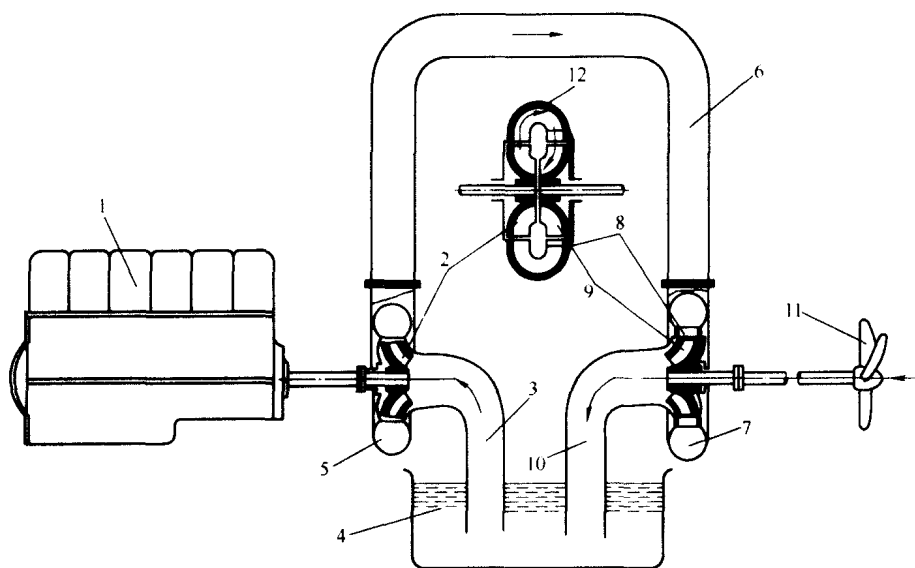
图 0-1 液力传动原理
