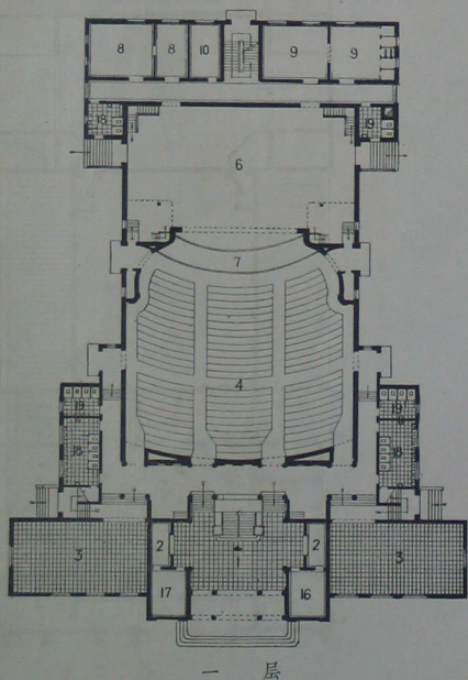
一 层
