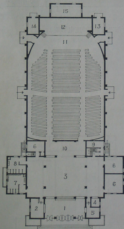
一 层 平 面
