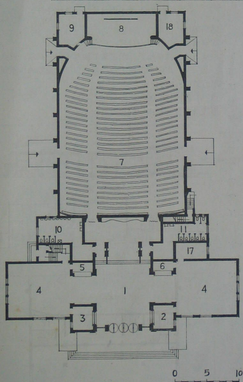
一层平面
