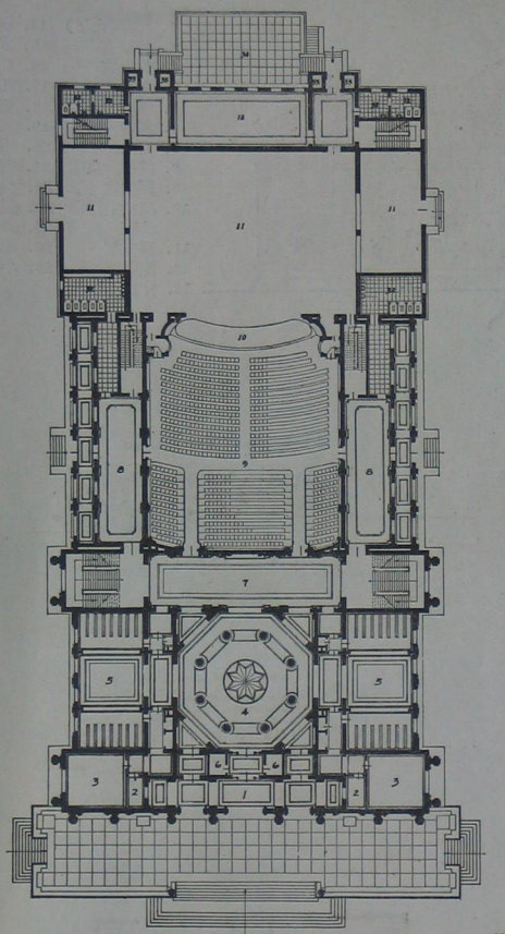
一 层
