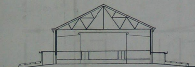
橫剖面
