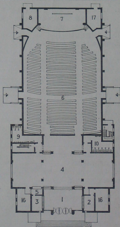
一层平面
