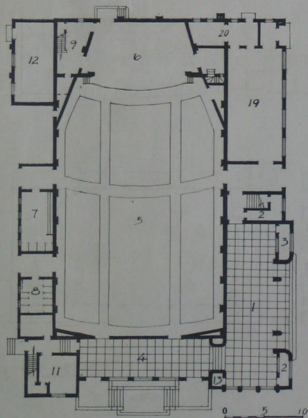
一 层
