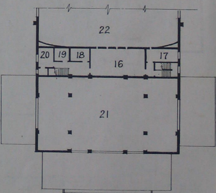
二 层 平 面
