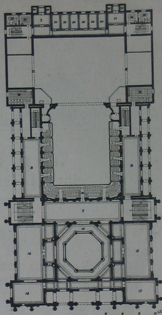
二 层
