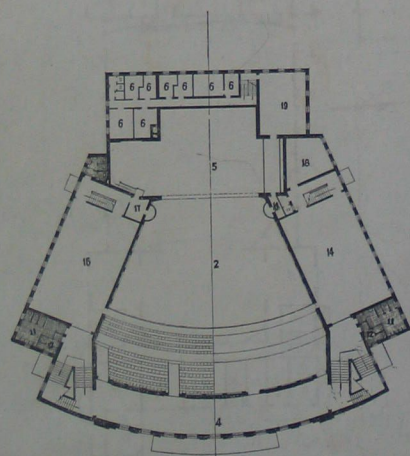
二 层
