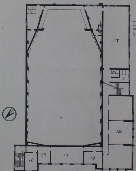
二 层
