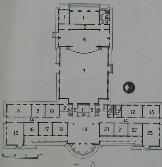
一层
