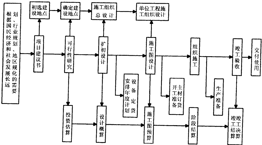
图 1-1 工程建设程序
