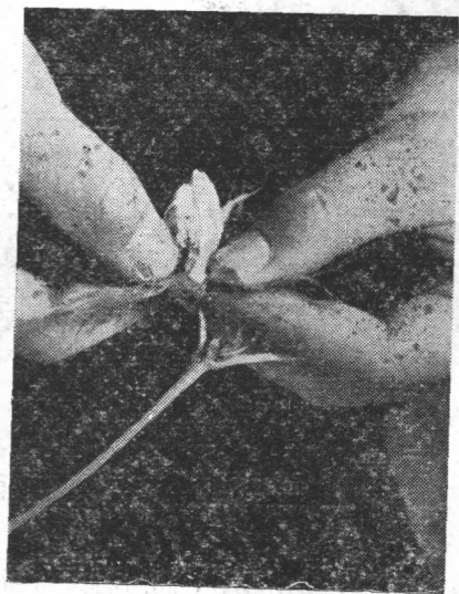
去勢時剝花的手勢、部位及剝破花冠與雄蕊管的情形
