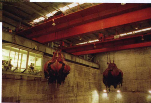
▲ 垃圾自动搬运系统
