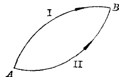
图 1-3 内能变化与途径无关
