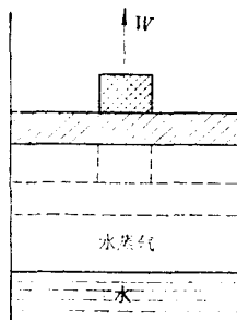
图 1-4 体系吸热作功示意图
