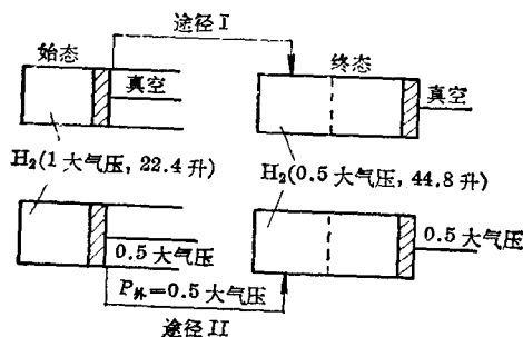
图 1-2 不同途径膨胀的功和热示意图
