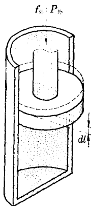
图 1-1 气体膨胀对外作功示意图
