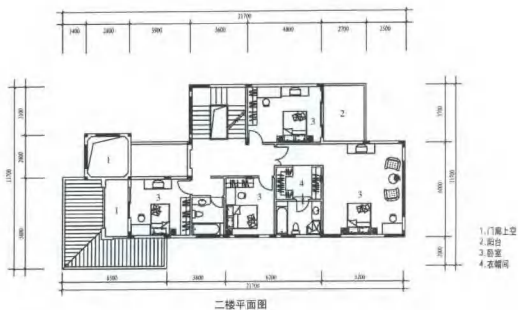
二樓平面圖
