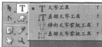
图 1-12 文字工具组
