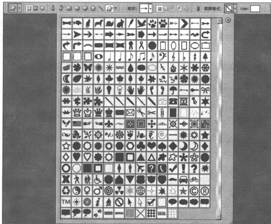
图 1-15 形状面板
