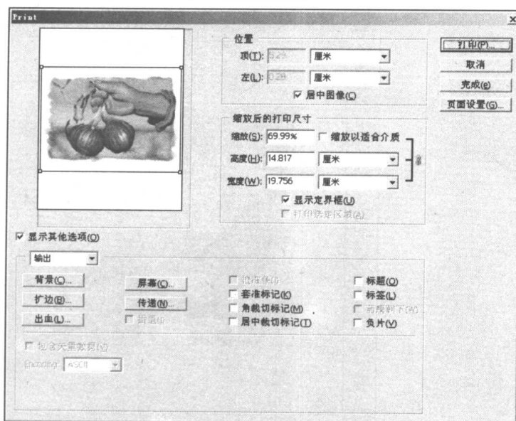
图 1-22 Print 对话框
