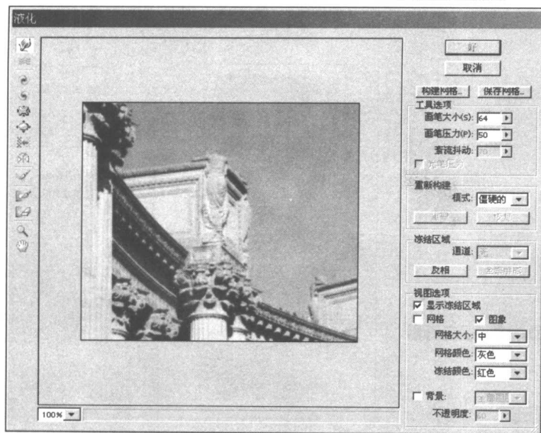
图 1-19 【液化】对话框
