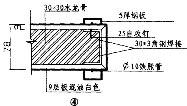
影视架剖面图
