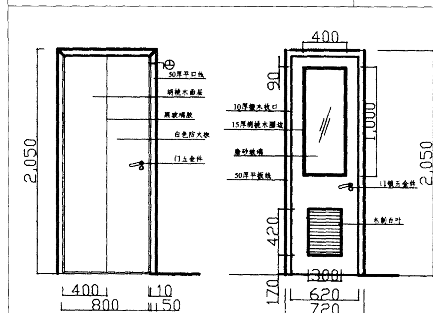
卧室门立面图
