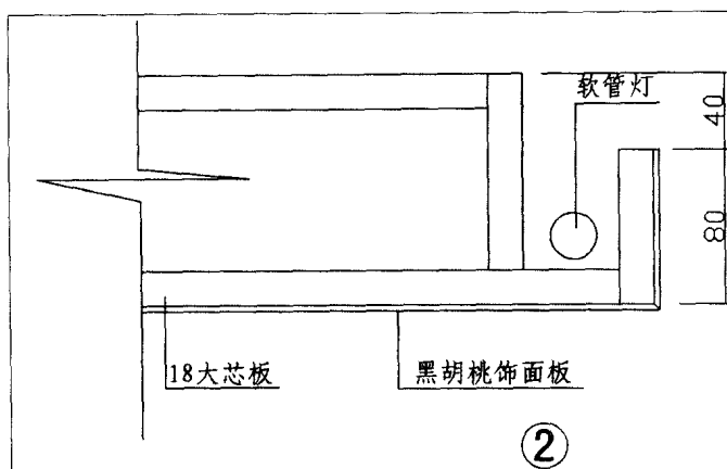
餐厅吊顶剖面图
