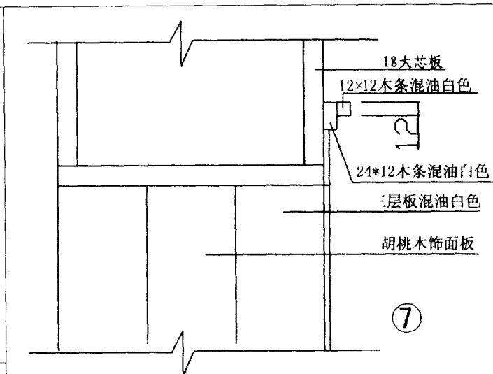
亚口剖面图
