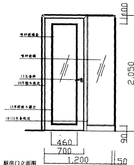
厨房门立面图
