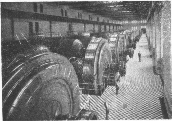
所電發之騰哈爾羅托 二十
