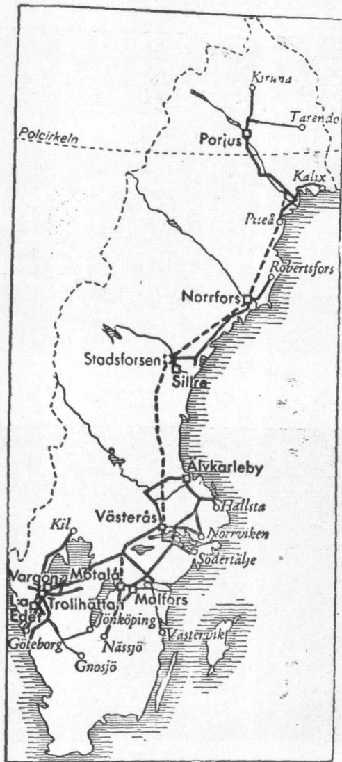
十 國電業主之幹傳線路虛線示將來建設計劃
