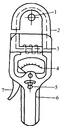
图 1-3 钳形电流表的外形图
