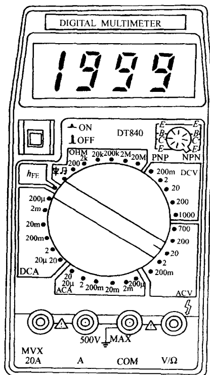
图 1-2 DT840 数字式万用表的面板结构图
