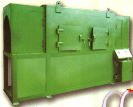
鋼管道在線拋丸除銹機
