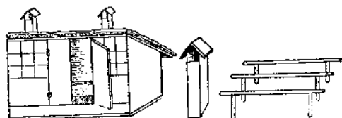
圖 6 改造後——前高後低，設簡單通風筒，合理的棲架
