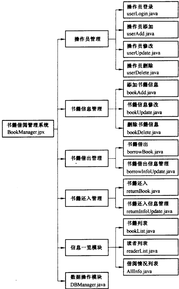
图 3-1 书籍借阅管理系统总体结构
