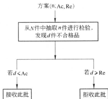
图 1-1 计数型抽样方案框图
