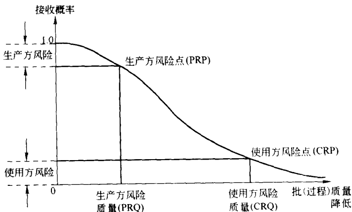
图 1-2 由生产方风险质量 (PRQ) 和使用方风险质量 (CRQ) 确定的 OC 曲线
