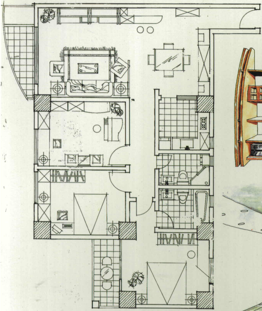
三室一厅平面布置图
