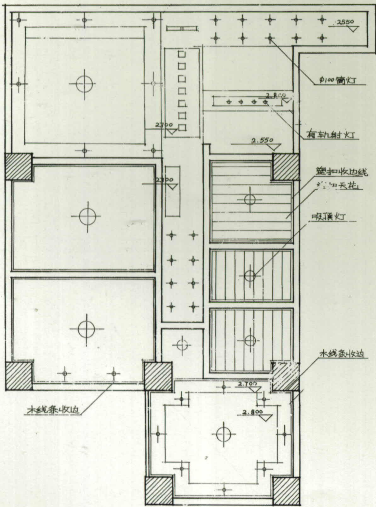
A型住宅吊顶平面图 1:50
