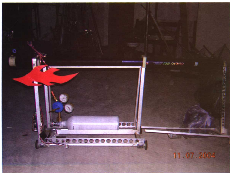
24、固若金汤——防干扰机器人“飞火”
