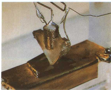
◎贝尔实验室的第一根晶体管
