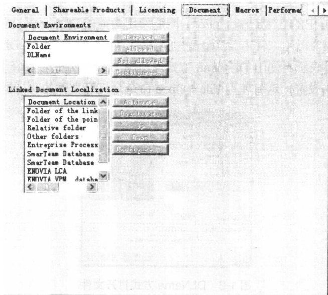
图 1-6 Document 选项卡
