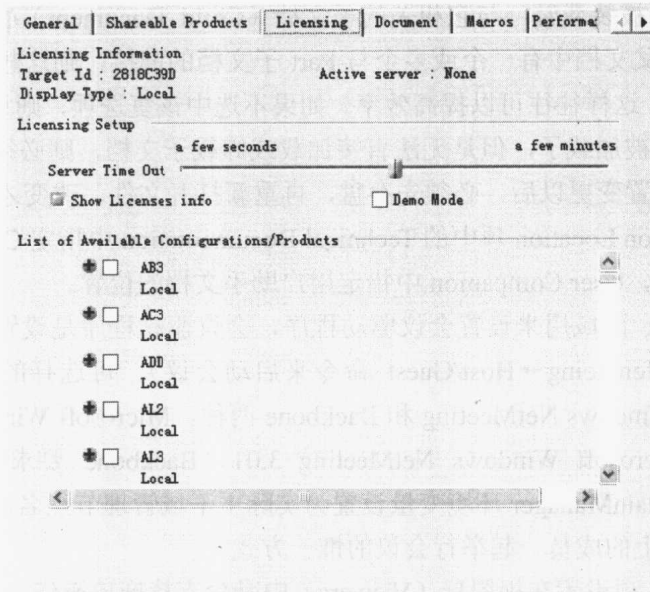
图 1-5 Licensing 选项卡
