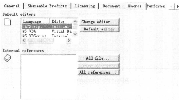
图 1-10 Macros 选项卡
