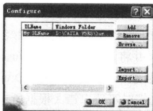
图 1-7 设置 DLName
