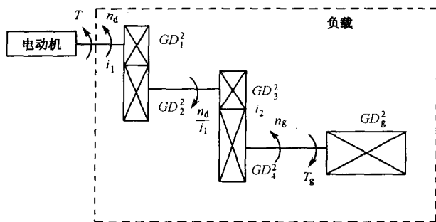
图 2.2 多轴电力传动系统
