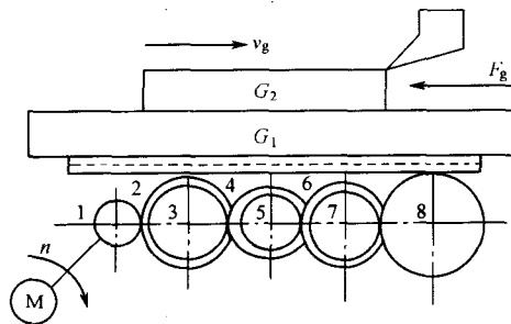
图 2.3 刨床传动系统示意图
