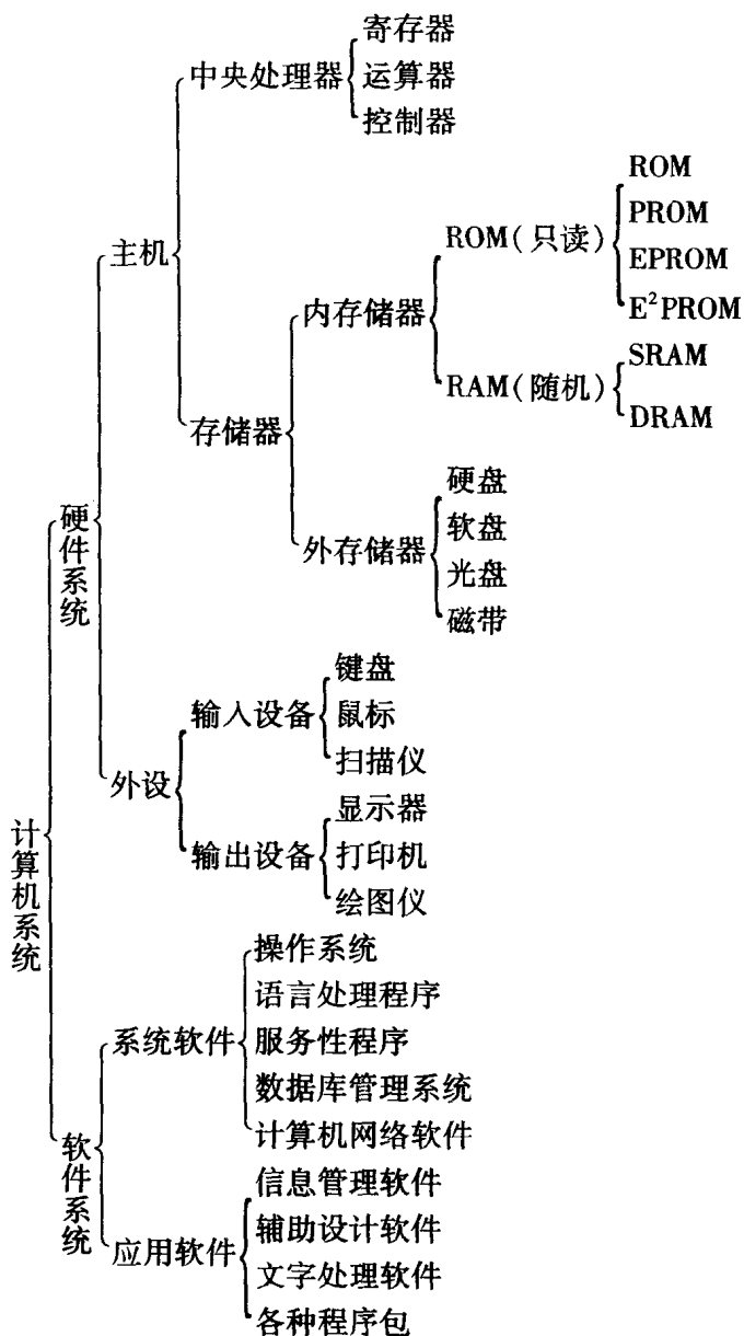
图 1-1 计算机系统的组成结构
