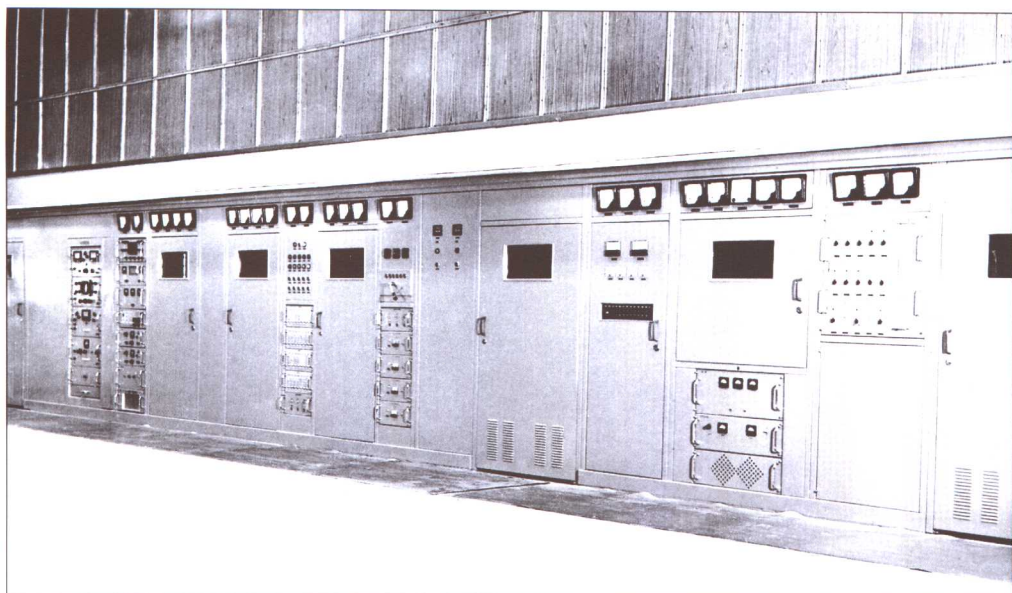
1969年，北京广播器材厂研制的 中国第一部特大功率1000千瓦短波广 播发射机
