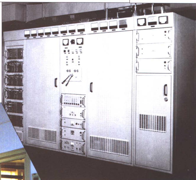
1973年至1974年，北京 广播器材厂研制成功中国第 一部甚高频三波段(6至12频 道)10千瓦中频调制彩色电视 发射机
