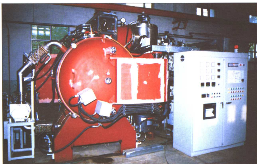
1998 年, 北京建中机器厂研制的 HVF6090GQ (L1211 II -4/ZM 型) 一次封排炉
