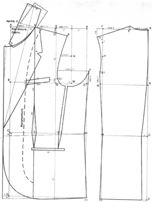
西服衣身的平面结构
