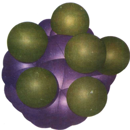
图 5 C_{60}Cl_6 化合物, C_{60} 开创了有机化学的新篇章。
