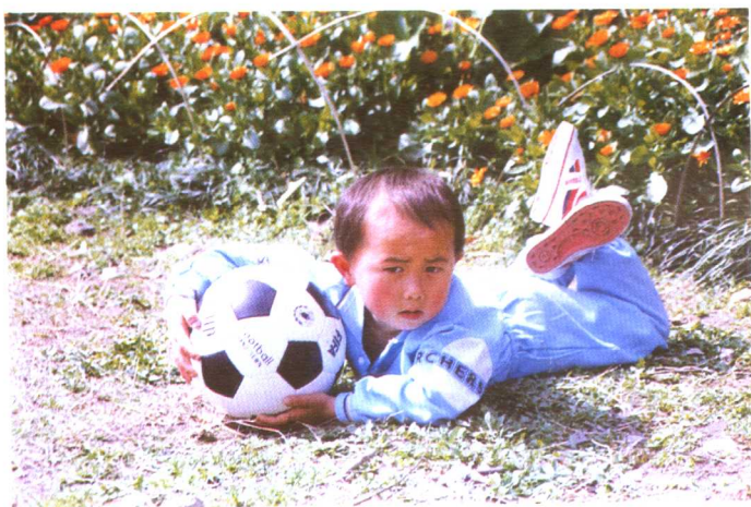
图2 足球,它由十二个五边形(黑色)和二十个六边形(白色)拼成。 C_{60} 分子的结构与它相似。
