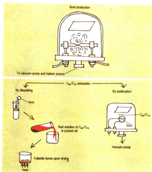
图 3 C_{60}/C_{70} 固体的制备。
