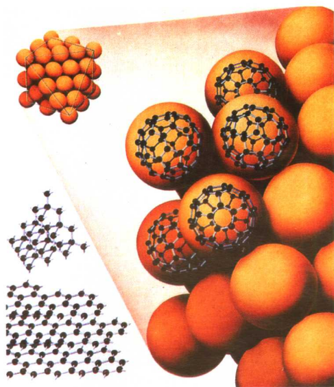
图1 固体碳的三种形态
