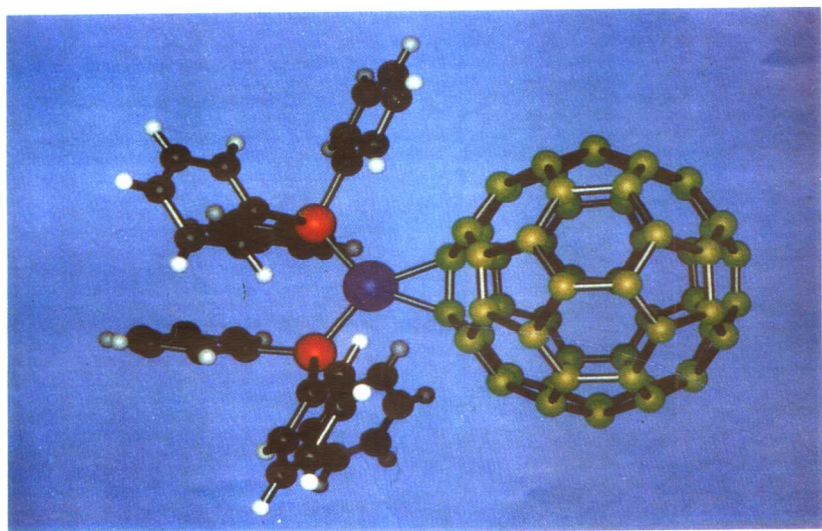
图 6 [(C_6H_5)_3P]_2Pt(\eta^2-C_{60}) 化合物, 绿色和黑色为碳原子, 蓝色、红色和白色分别为铂原子、磷原子和氢原子。
