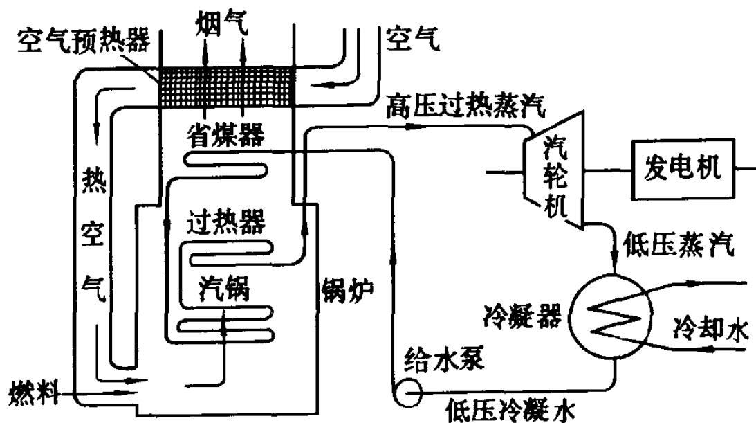
图 0-1 简单蒸汽动力装置示意图
