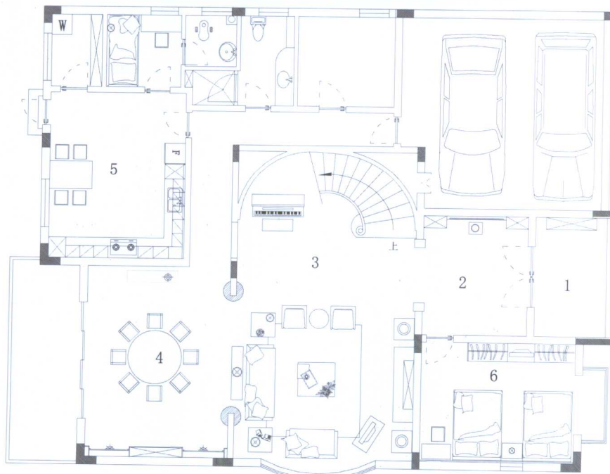
一层平面布置图
