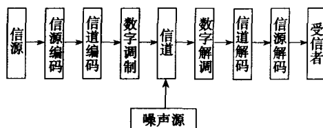
图 1-2 数字通信系统的基本模型
