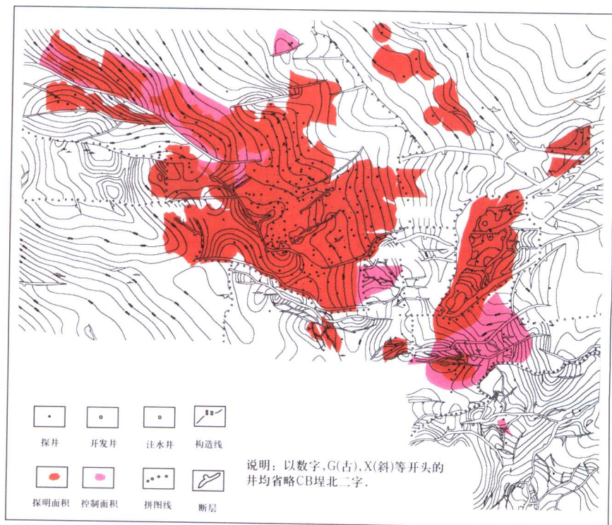
埕岛油田构造井位图
