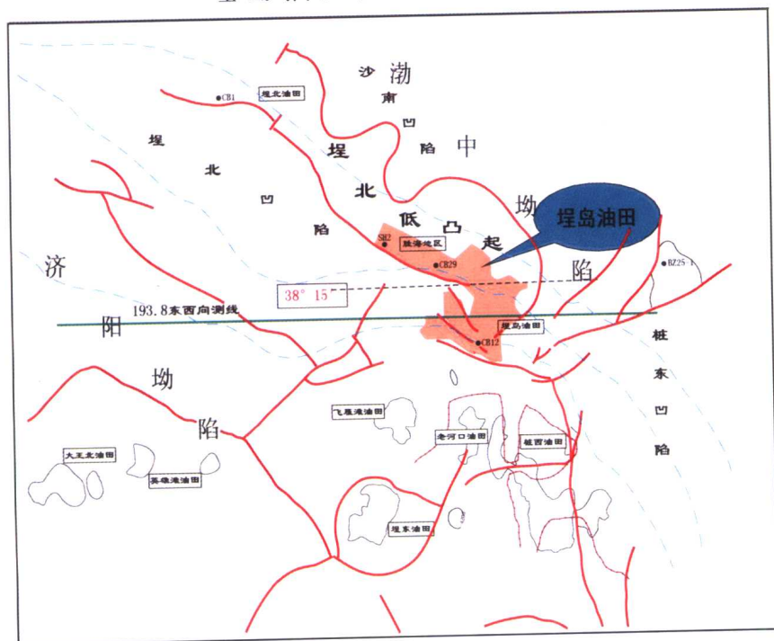
埕岛油田区域构造位置图
