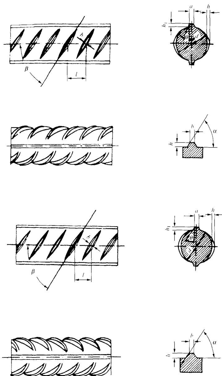
d —钢筋内径; \alpha —横肋斜角; h —横肋高度; \beta —横肋与轴线夹角; h_1 —纵肋高度; \theta —纵肋斜角; a —纵肋顶宽; l —横肋间距; b —横肋顶宽
