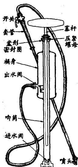
WD-0.55型单管喷雾器结构图
